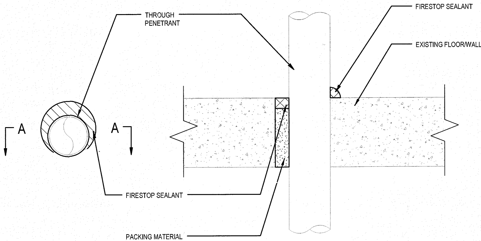
SECTION A-A
